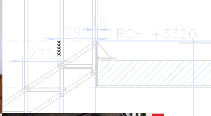
Mittelholmtreppe Privathaus Velbert 2005 Stufen Buche gebeizt
